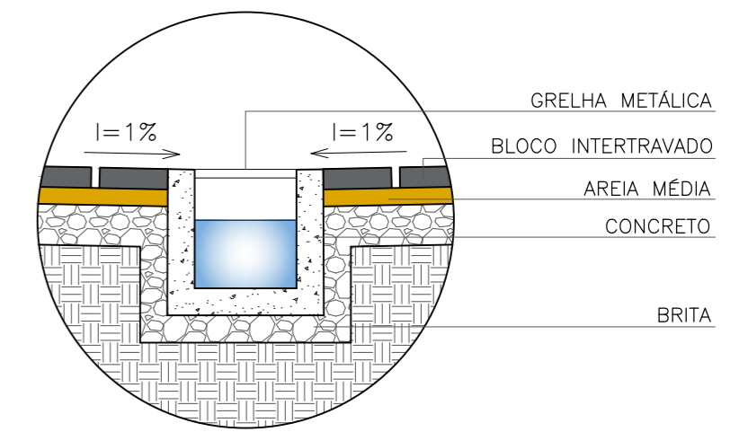
DETALHE CANALETA C/ GRELHA METÁLICA CORTE ESC. 1:20
