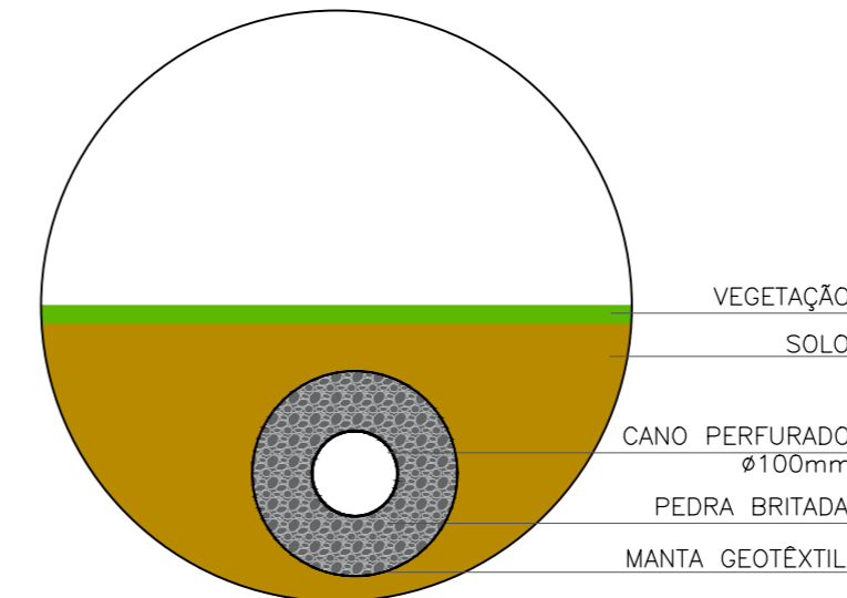
DETALHE DRENO CORTE ESC. 1:10
